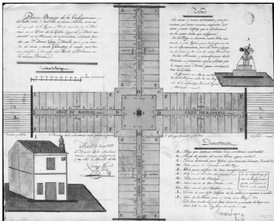
Lám. 3. Lámina de la configuración de Santa Amalia (Año 1826).
