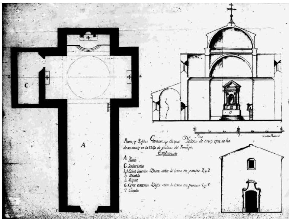
Lám. 4. Planta y alzado de la iglesia parroquial de Santa Amalia.
