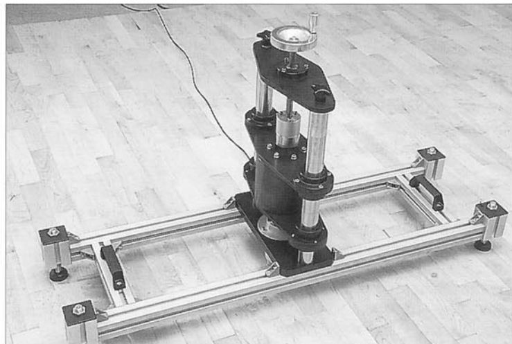
El servicio de pavimentos deportivos del IBV incluye la realización de los ensayos más importantes de la normativa internacional.
